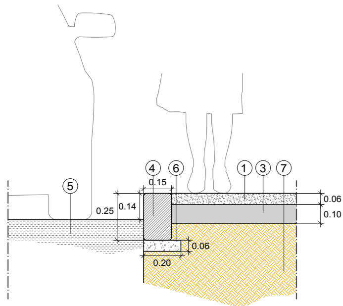
DETALLE 1 CALZADA-TERRIZO PARA PEATONES
